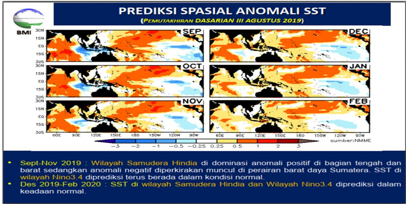
Gambar 4.1 prediksi SST
