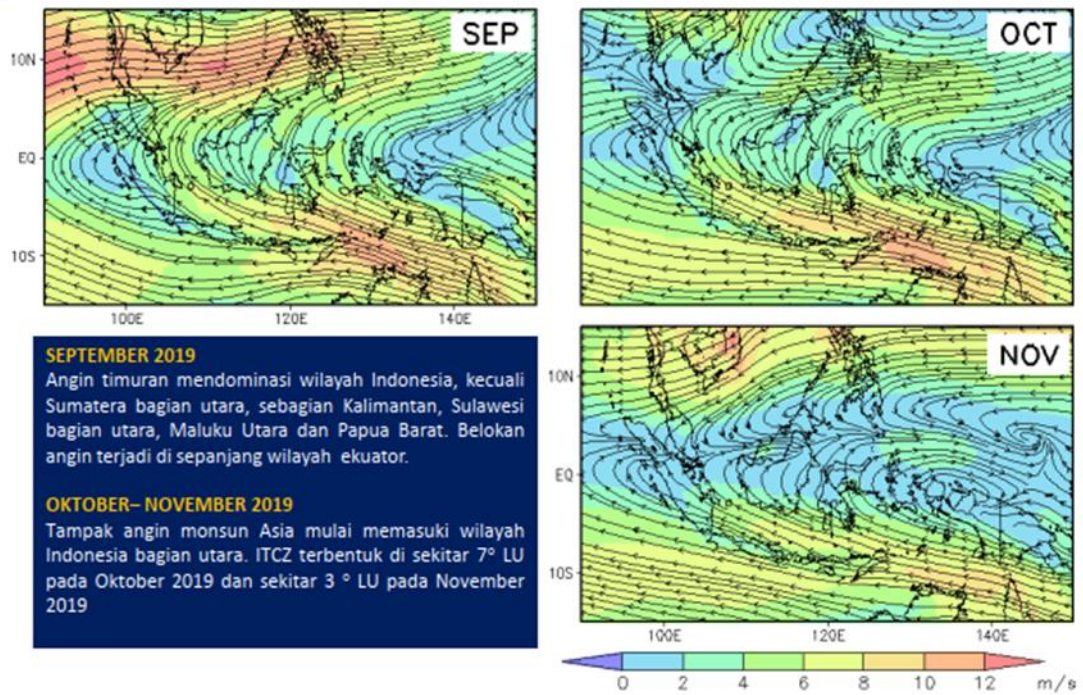
Gambar 4.3 ANGIN LAPISAN
